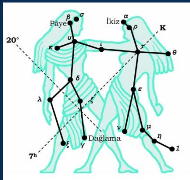
İkizler Takımyıldızı
