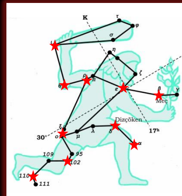
Herkül Takımyıldızı
