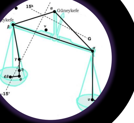
Terazi Takımyıldızı
