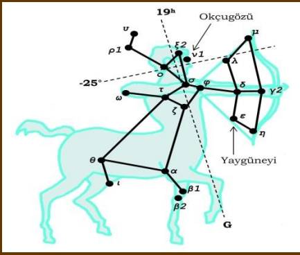
Yay Takımyıldızı
