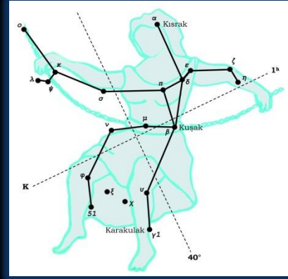
Zincirli Prenses
