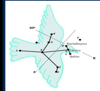
Kartal Takımyıldızı
