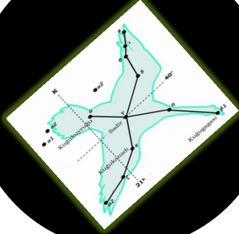
Kuşu Takımyıldızı
