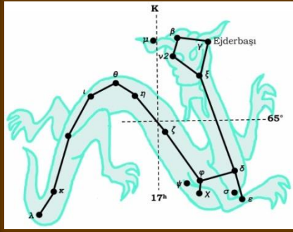
Ejderha Takımyıldızı
