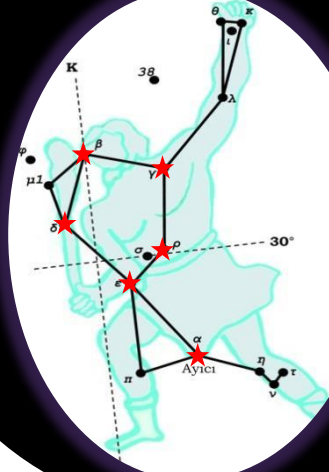
Çoban Takımyıldızı
