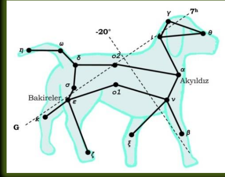
Büyük Köpek
